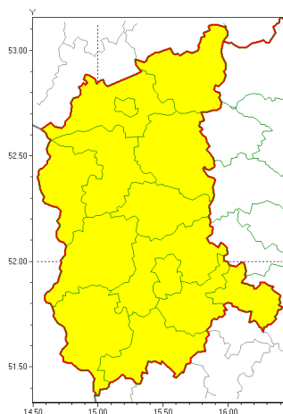
Silny wiatr 2019-09-17 06:59
